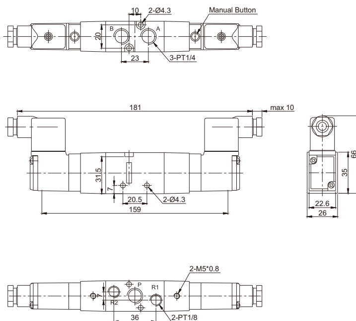
TVF3 3 / 4 30-□D/DZ-02
