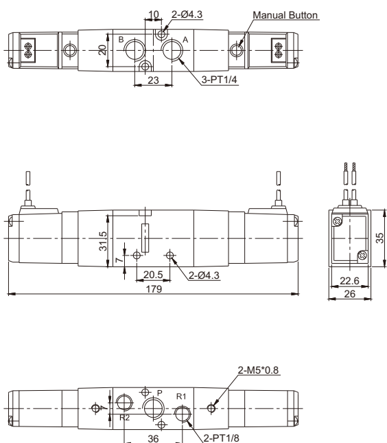
TVF3 3 / 4 30-□G-02
